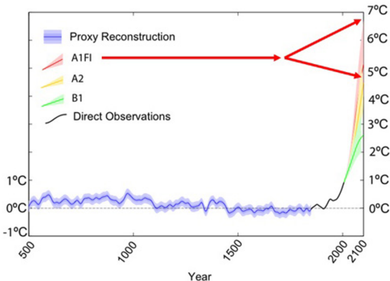
Fig. 1: Temperaturas globales comparadas con 1800-1900 según diferentes escenarios de emisiones del IPCC. Durante la última década las emisiones de CO 2 se han movido por el “peor escenario” definido en 2000, el “A1 FI”, que nos llevaría a un calentamiento global de entre 5 a 7° aproximadamente. Fuente: IPCC, 2001
