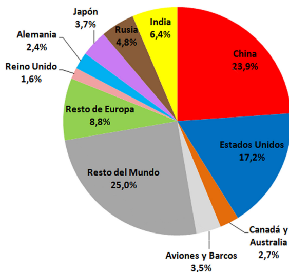
Gráfico 1: Emisiones actuales y acumuladas de dióxido de carbono causado por combustibles fósiles (Hansen 2009: 189, gráfico actualizado en el internet 1 )
