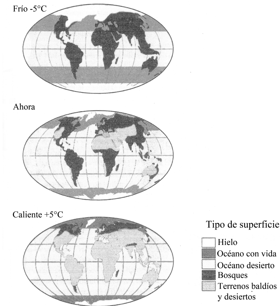
Gráfico 5: La distribución de la vida hoy y en un planeta más frío o más caliente (Lovelock, 2007: 101 modificado)
