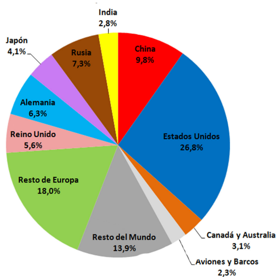
Gráfico 1: Emisiones actuales y acumuladas de dióxido de carbono causado por combustibles fósiles (Hansen 2009: 189, gráfico actualizado en el internet 1 )
